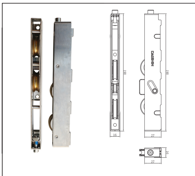
Bánh xe 2 bánh hệ 120
