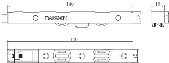
Bánh xe thấp 2 bánh 80
