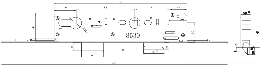
Thân khóa đa điểm XINGFA Mã : DA8530
