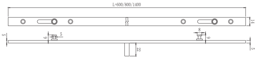
Thanh chuyển động nhôm cửa lùa Mã:DACL600, DACL1400
