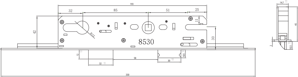
Thân khóa đơn điểm XINGFA Mã: DAD8530
