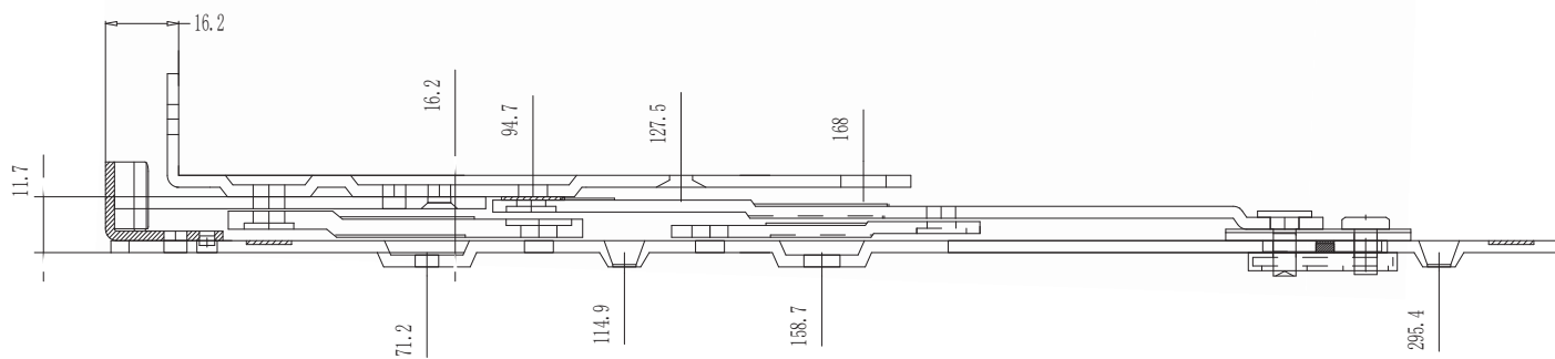
Bản lề chữ A mở quay 13 inch rãnh 13.5 (chịu lực) Mã: DAEL13.5-13
