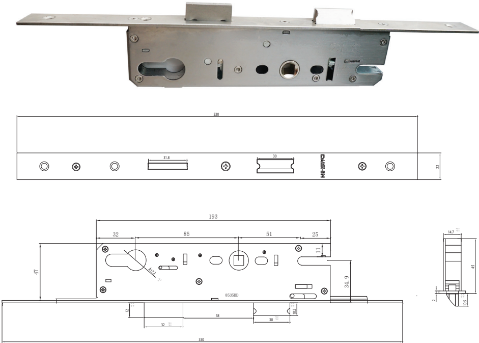
Thân khóa đơn điểm Châu Âu Mã: DAD8535
