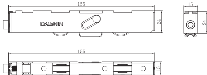
Bánh xe cao 2 bánh 80
