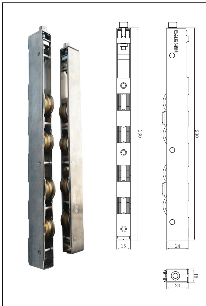
Bánh xe cao 4 bánh 80
