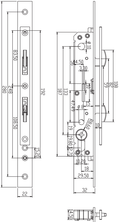
Thân khoá móc đôi 80
