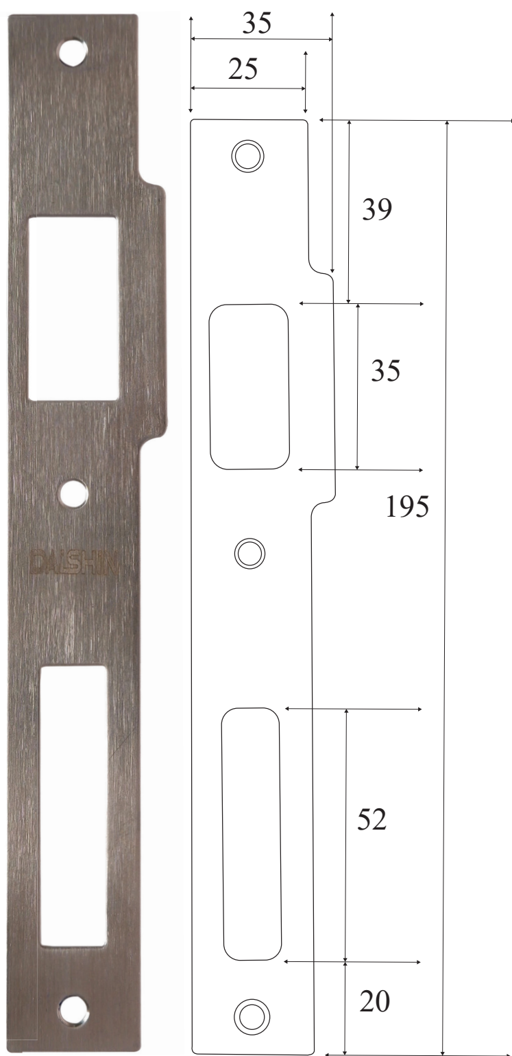
Miếng đôn khóa móc phẳng
