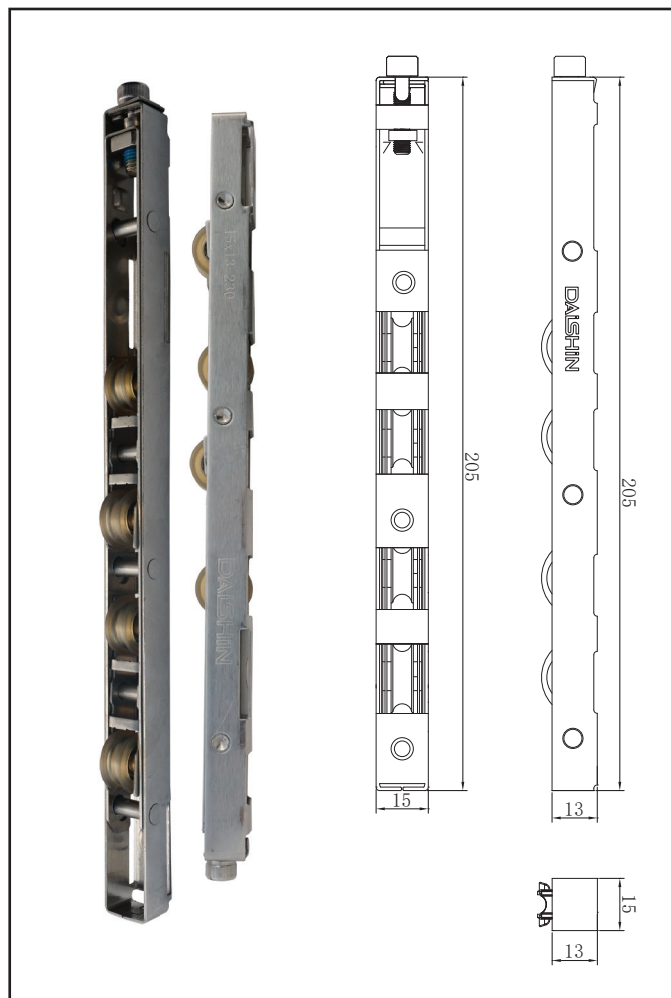
Bánh xe thấp 4 bánh 80
