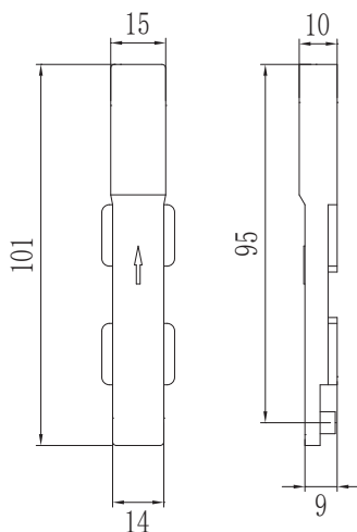
Đầu chốt cánh phụ 75
