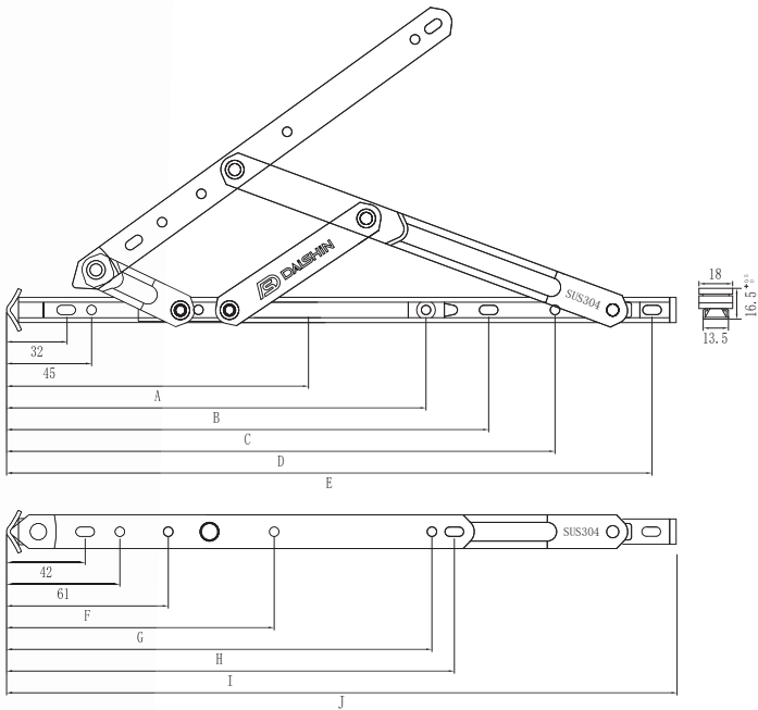
Bản lề chữ A mở quay rãnh 13.5
