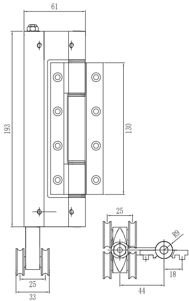
Bánh xe dưới xếp trượt 75
