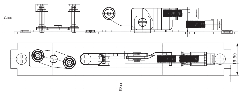
Bánh xe chống rung nhấc
