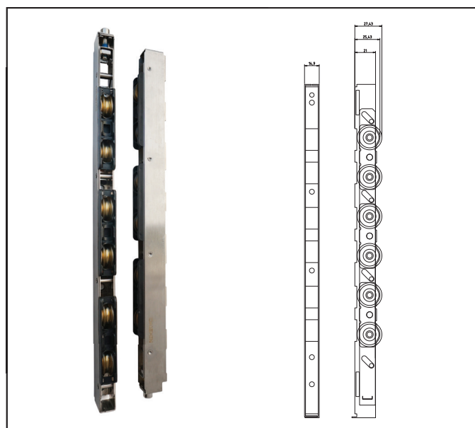
Bánh xe cao 6 bánh chống nhấc hệ 80
