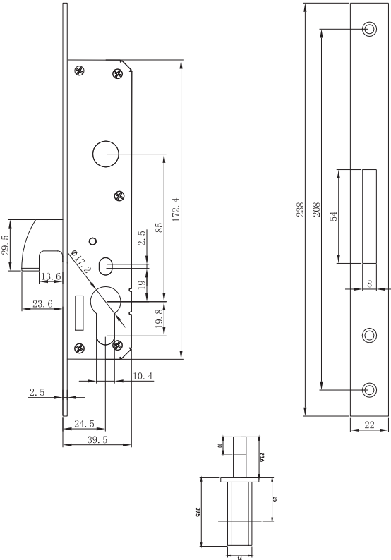
Thân khoá móc đơn 80
