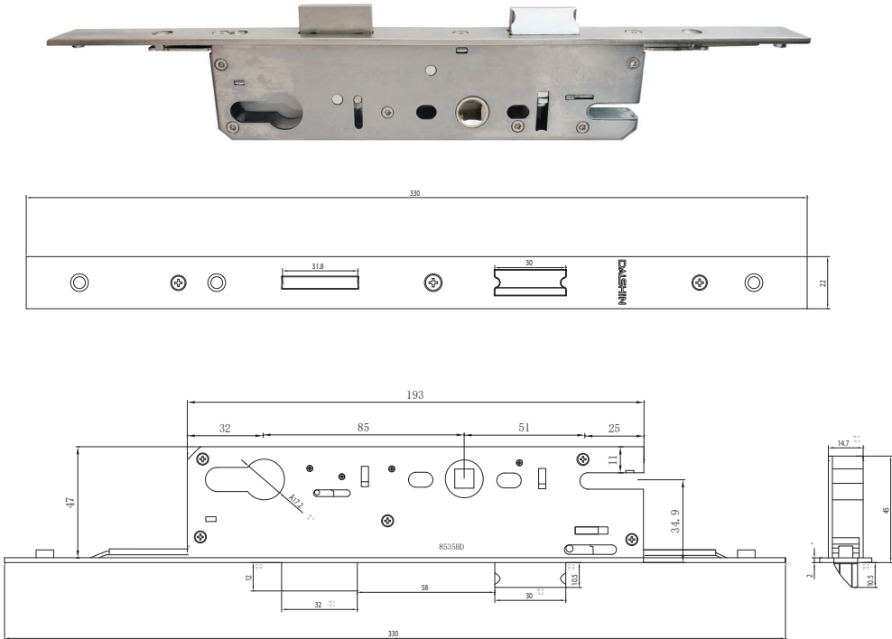
Thân khóa đa điểm Châu Âu Mã : DA8535
